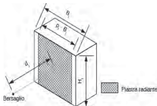
Illustrazione S.3-5 Schematizzazione della piastra radiante
