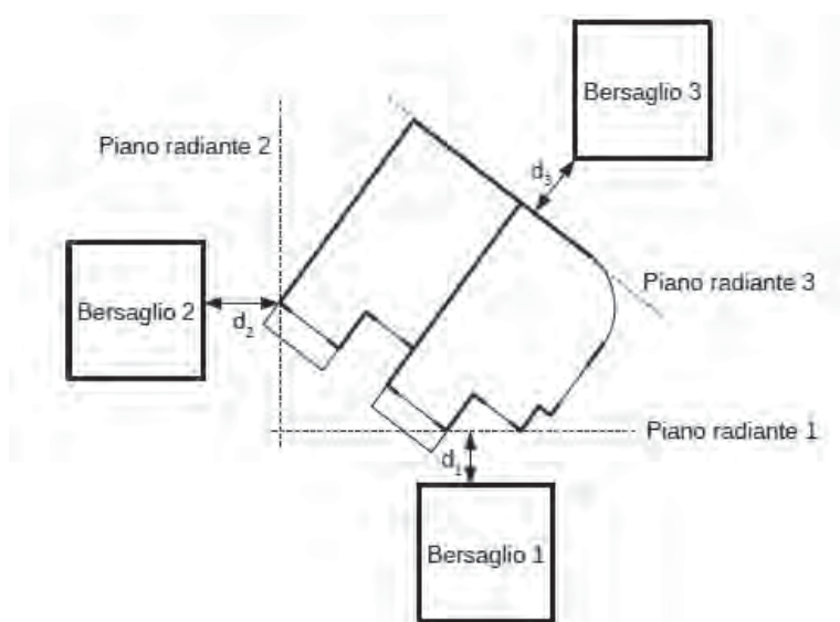
Illustrazione S.3-2: Determinazione del piano radiante, vista in pianta delle costruzioni.
