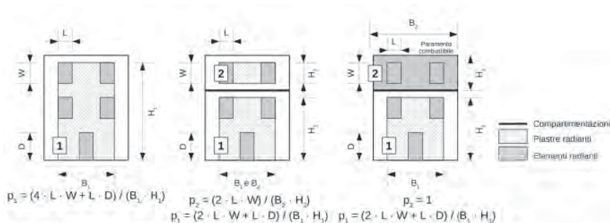
Illustrazione S.3-4: Esempio percentuale di foratura della i -esima piastra radiante, vista frontale
